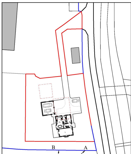
01 SITE PLAN 1:500
